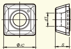
SPKX
