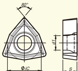
WCKX / WCMX
