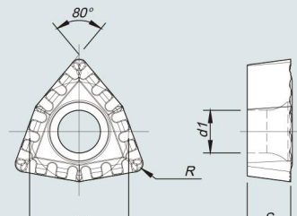
WCKX-LC
