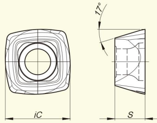
SPKW / SPKT
