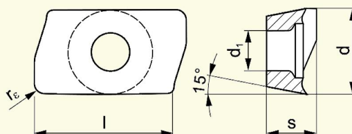
ADMX 11
